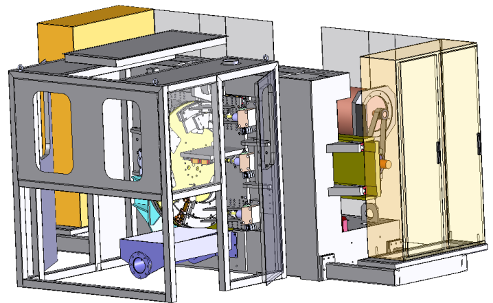
DDW neue Bauform Ausführung mit Transportscheibe (Pleuel)
