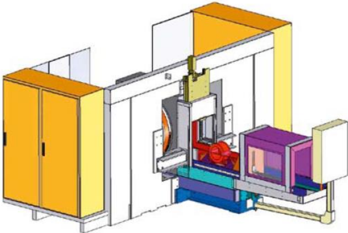
DDW neue Bauform Ausführung mit Werkstückschlitten
